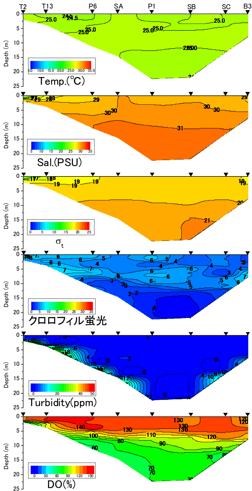
2013年9月29日における水温、塩分、密度 \sigma_t 、クロロフィル蛍光値、濁度、DO飽和度
