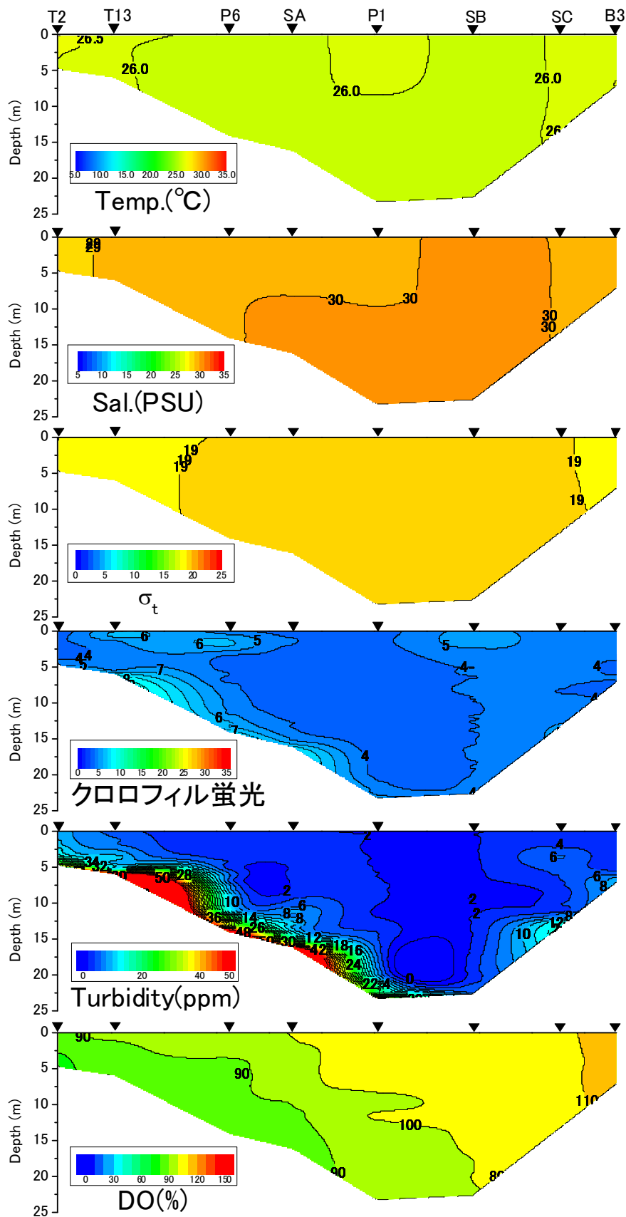
2013年9月23日における水温、塩分、密度 \sigma_t 、クロロフィル蛍光値、濁度、DO飽和度
