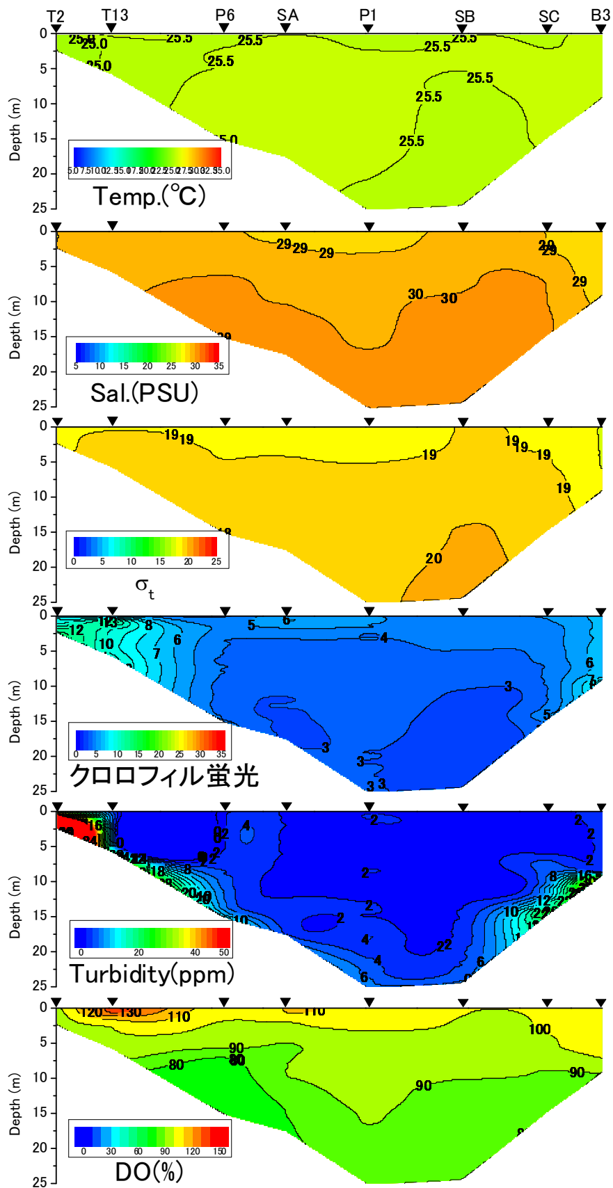
2013年9月18日における水温、塩分、密度 \sigma_t 、クロロフィル蛍光値、濁度、DO飽和度
