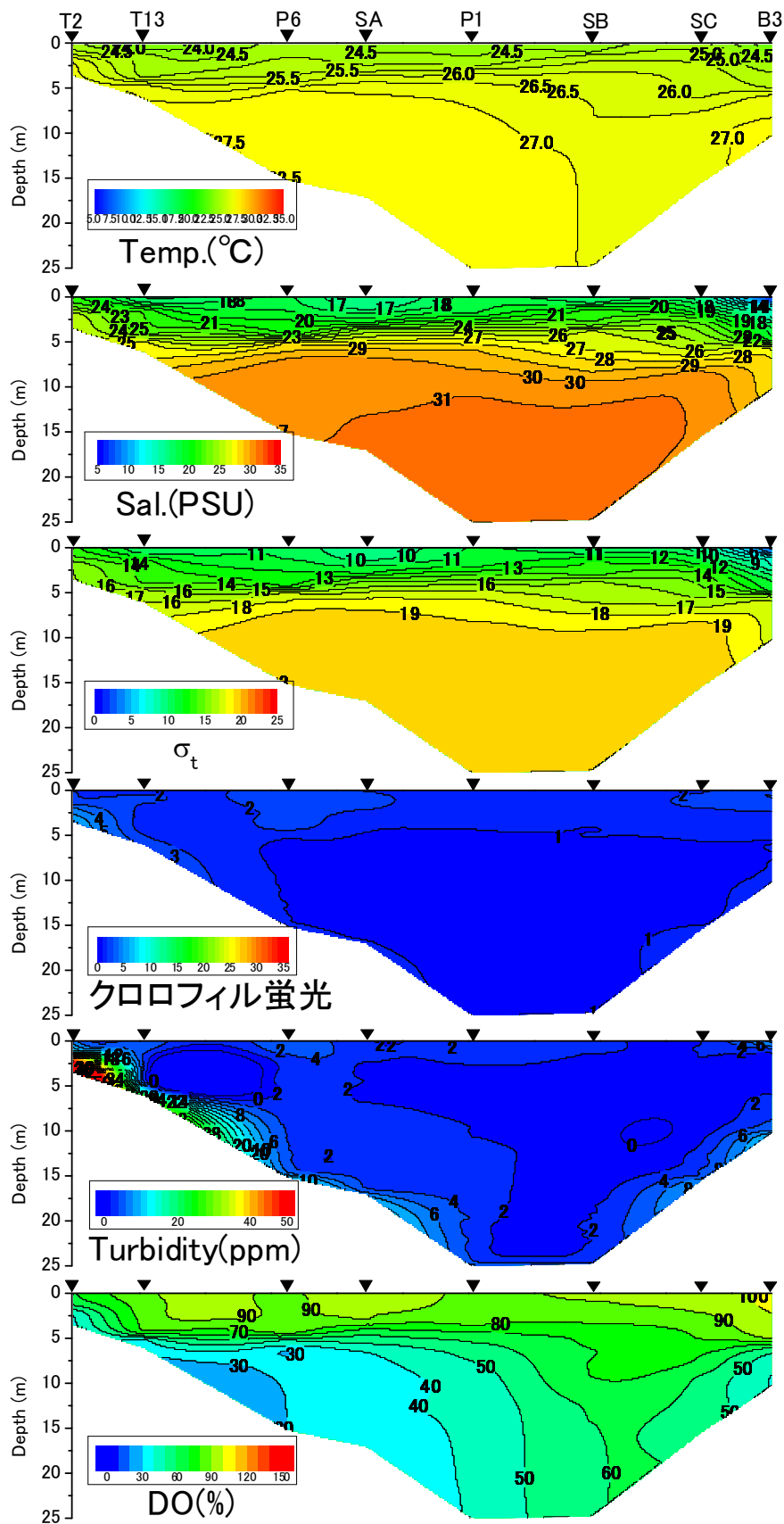
2013年9月5日における水温、塩分、密度 \sigma_t 、クロロフィル蛍光値、濁度、DO飽和度
