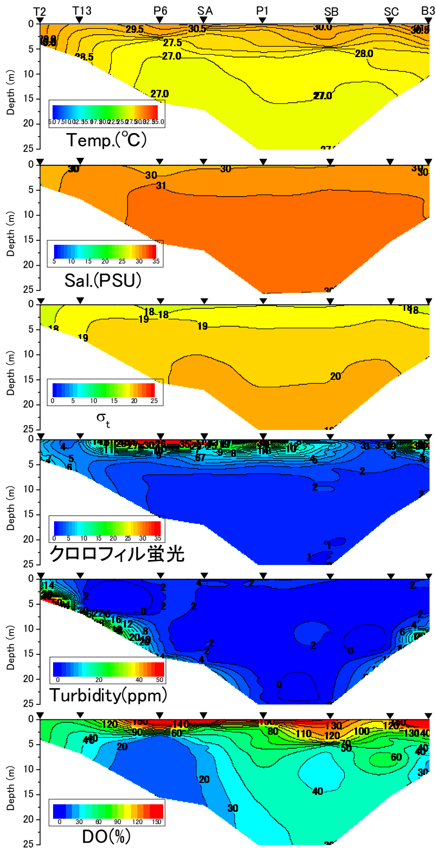
2013年8月21日における水温、塩分、密度 \sigma_t 、クロロフィル蛍光値、濁度、DO飽和度
