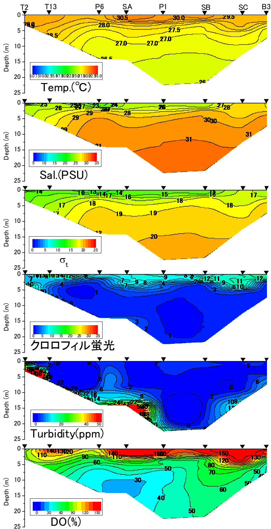
2013年8月8日における水温、塩分、密度 \sigma_t 、クロロフィル蛍光値、濁度、DO飽和度
