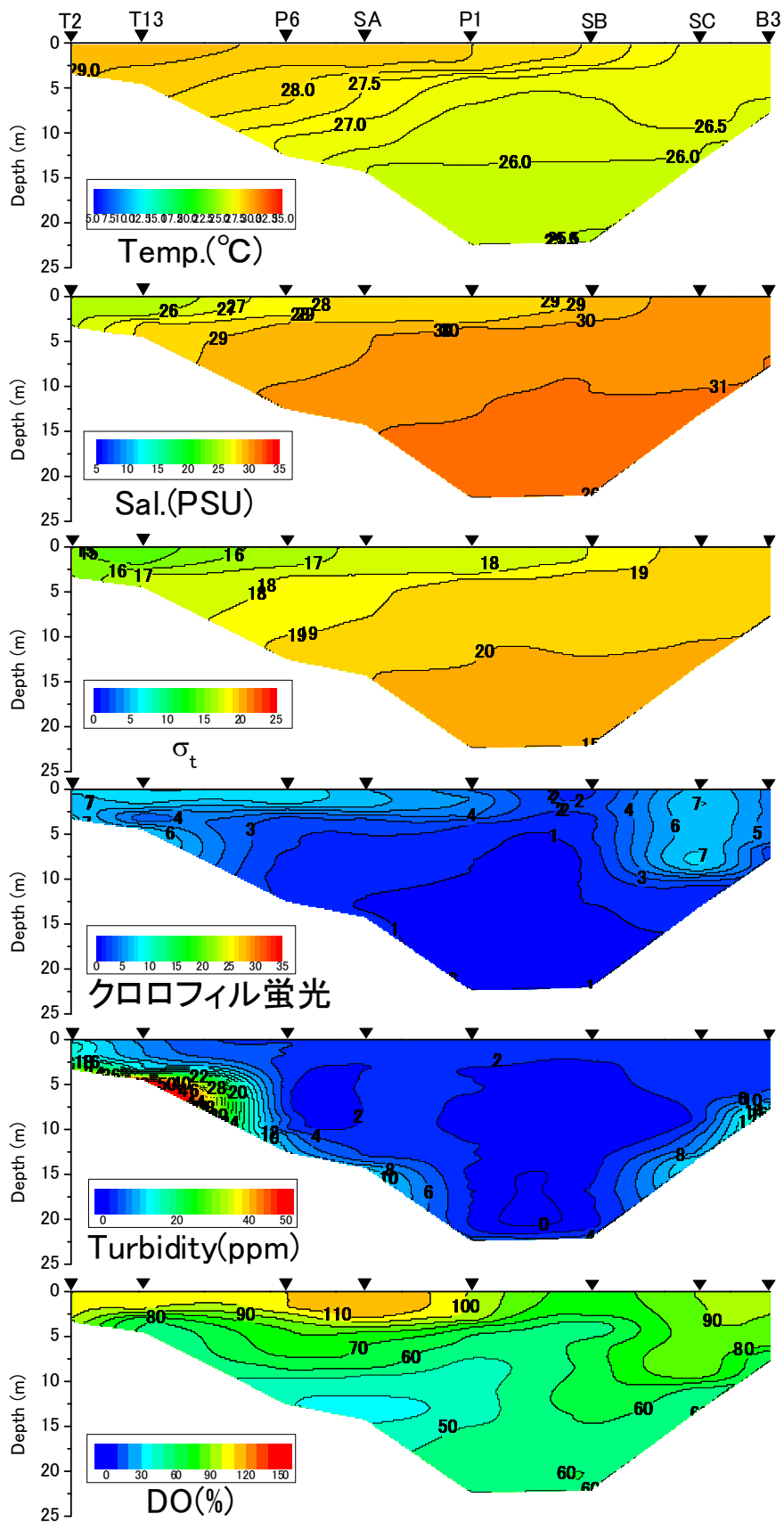
2013年7月31日における水温、塩分、密度 \sigma_t 、クロロフィル蛍光値、濁度、DO飽和度
