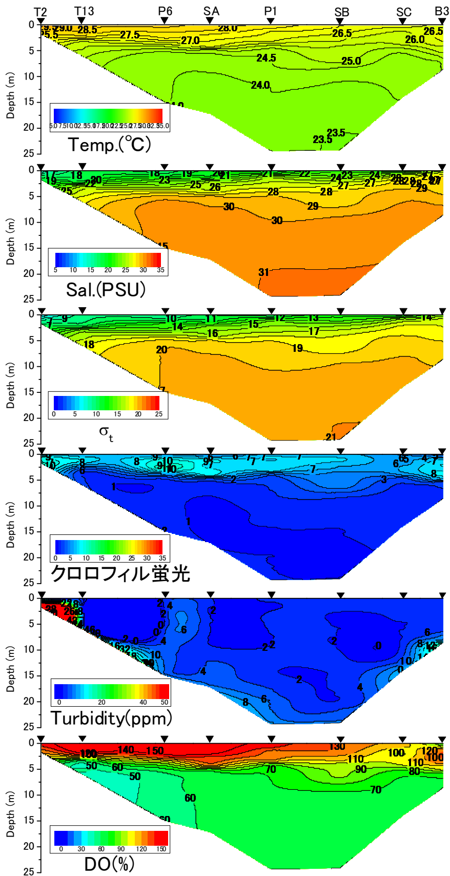
2013年7月10日における水温、塩分、密度 \sigma_t 、クロロフィル蛍光値、濁度、DO飽和度
