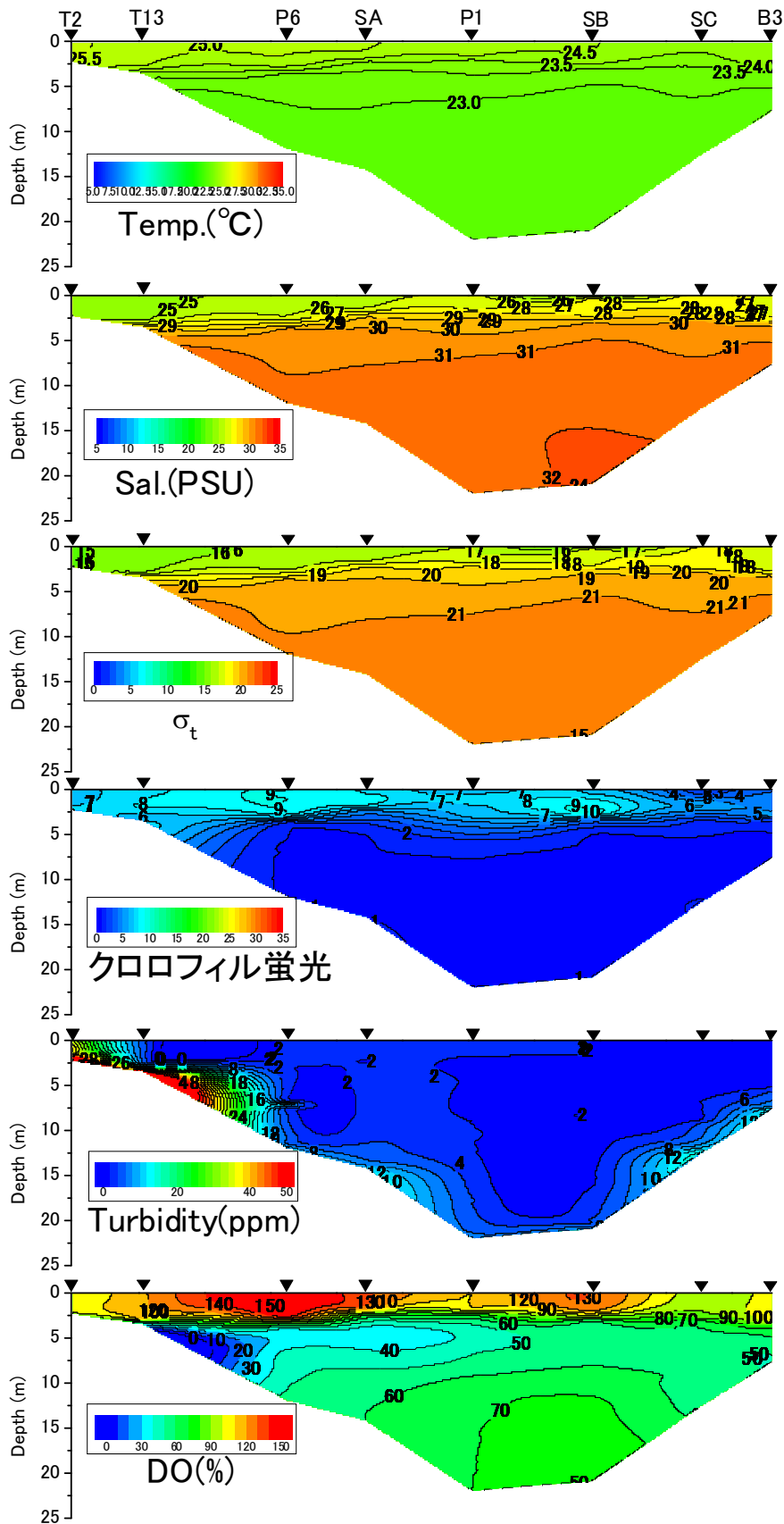
2013年7月2日における水温、塩分、密度 \sigma_t 、クロロフィル蛍光値、濁度、DO飽和度
