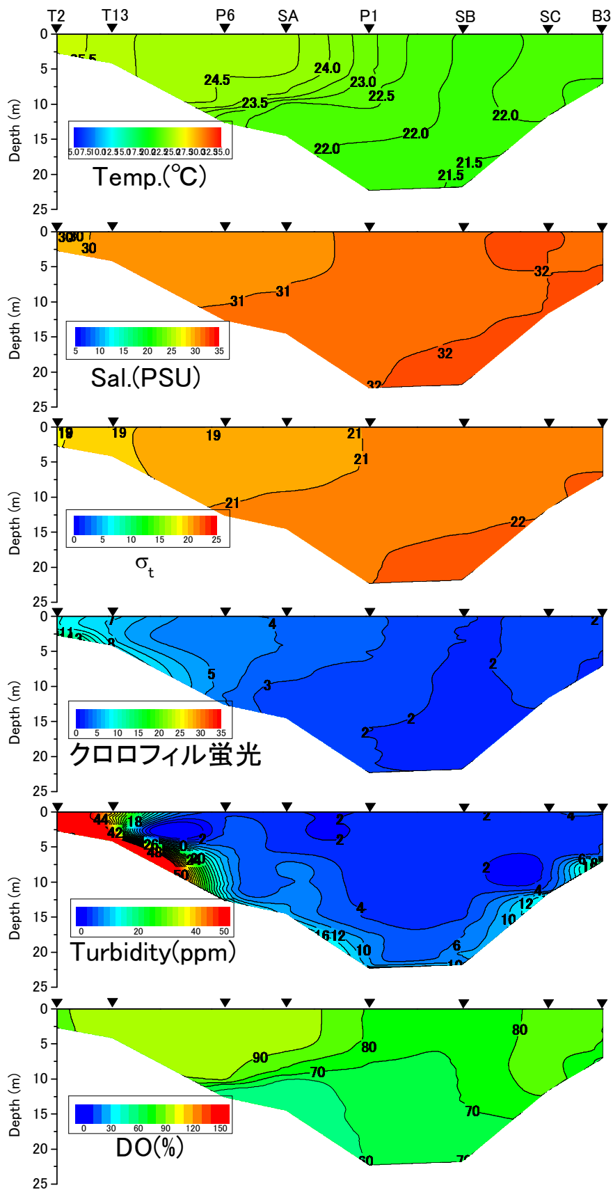
2013年6月19日における水温、塩分、密度 \sigma_t 、クロロフィル蛍光値、濁度、DO飽和度
