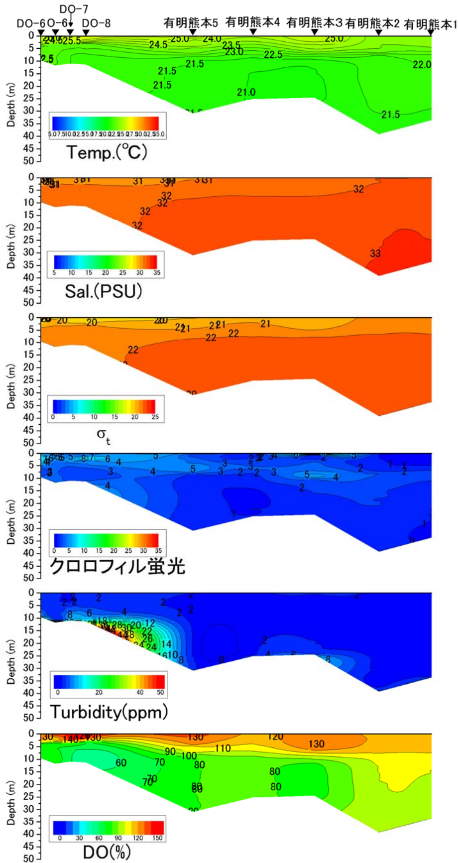
2013年6月17日における水温、塩分、密度 \sigma_t 、クロロフィル蛍光値、濁度、DO飽和度 (熊本県水産研究センター、西海区水産研究所観測)
