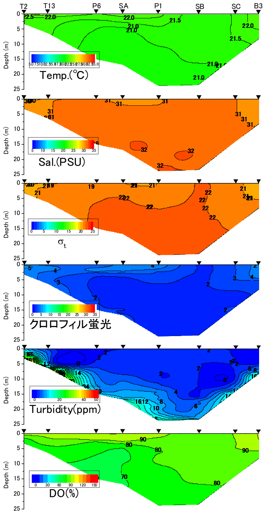
2013年6月11日における水温、塩分、密度 \sigma_t 、クロロフィル蛍光値、濁度、DO飽和度
