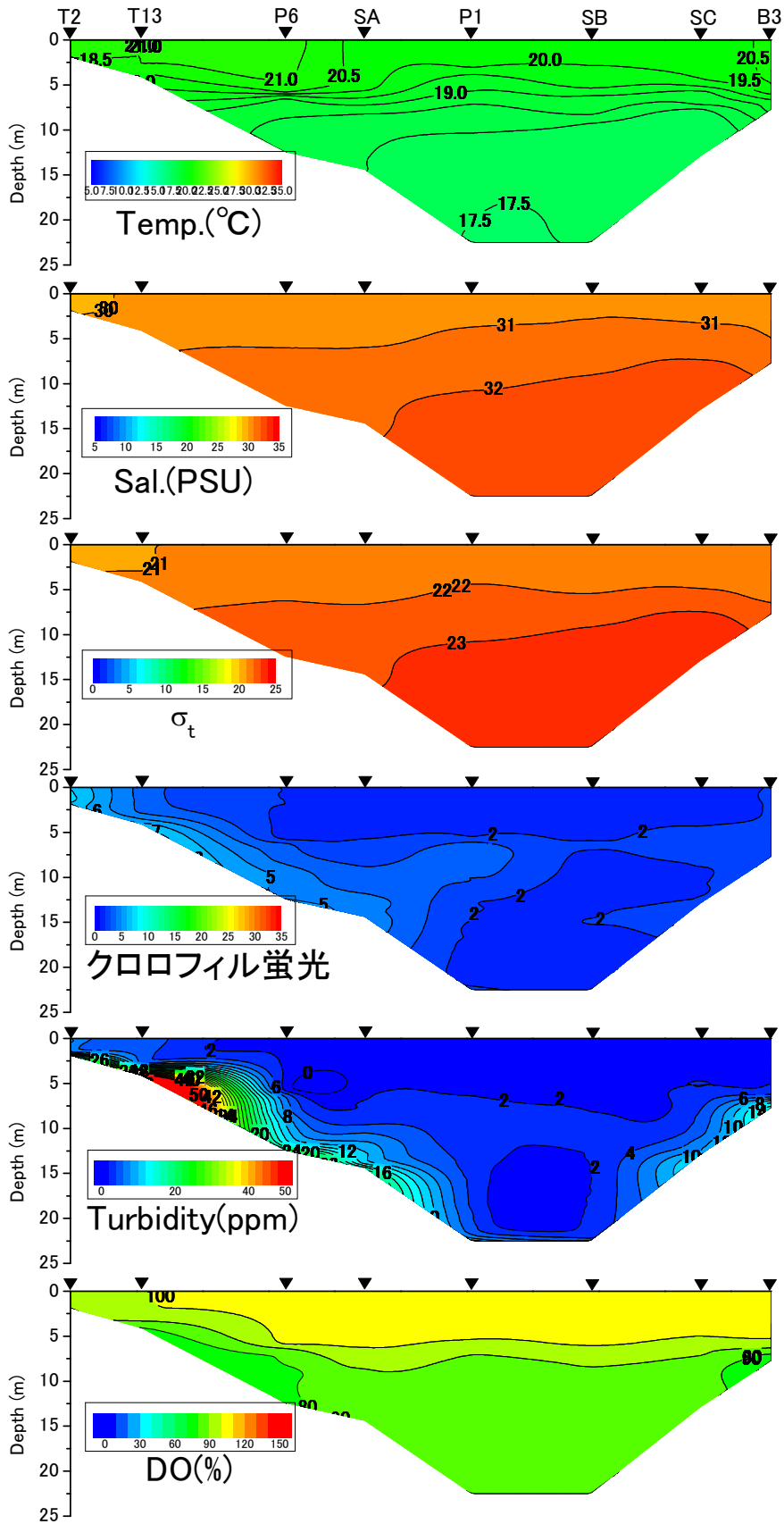
2013年5月19日における水温、塩分、密度 \sigma_t 、クロロフィル蛍光値、濁度、DO飽和度
