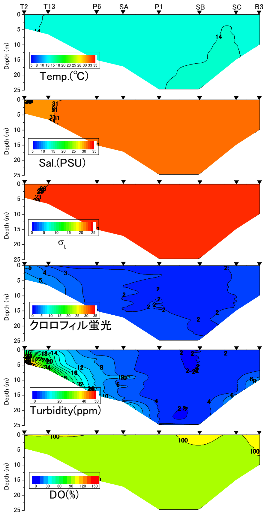
2013年4月11日における水温、塩分、密度 \sigma_t 、クロロフィル蛍光値、濁度、DO飽和度
