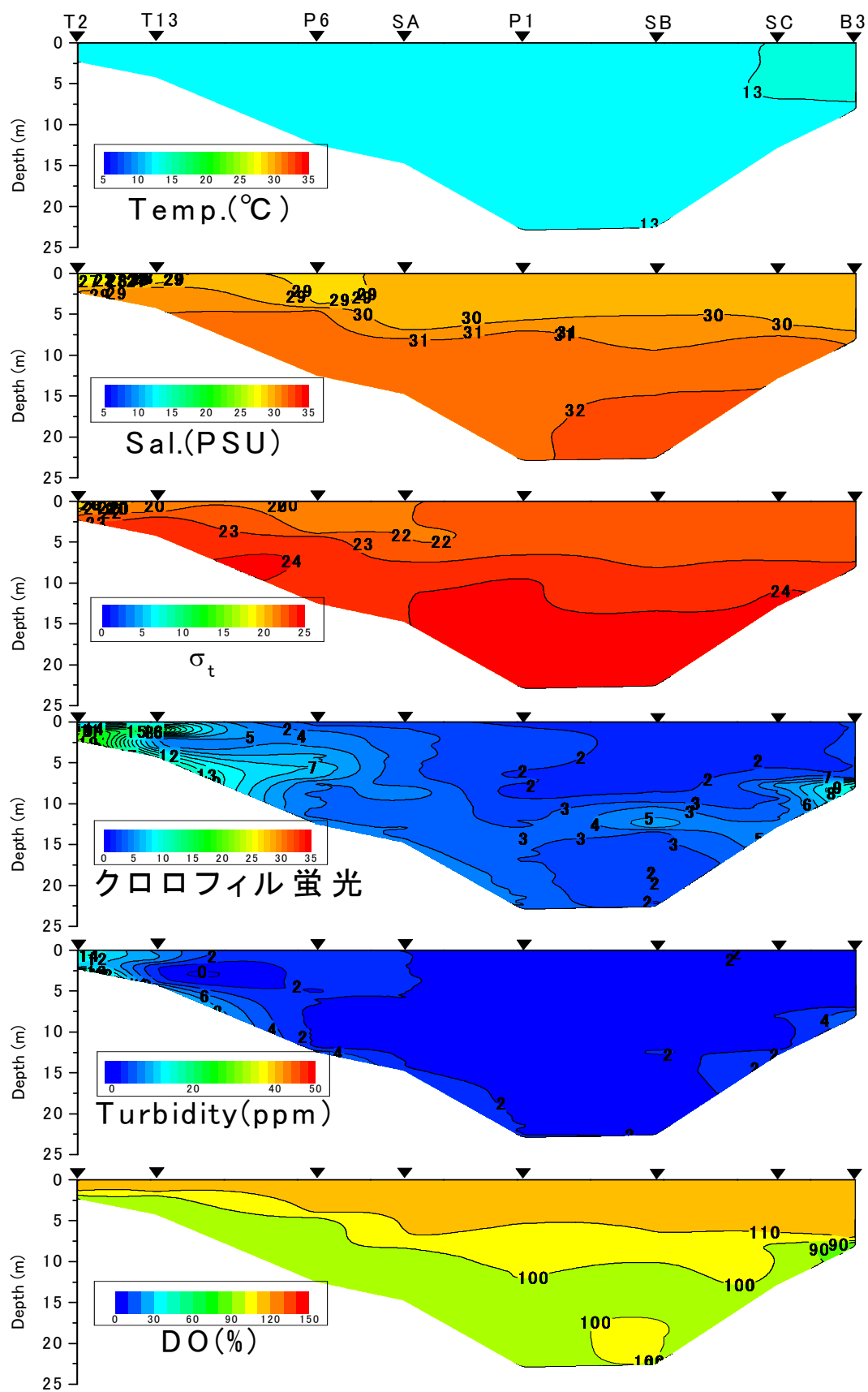
有明海湾奥西部海域の水質の断面分布（2013年3月21日）
