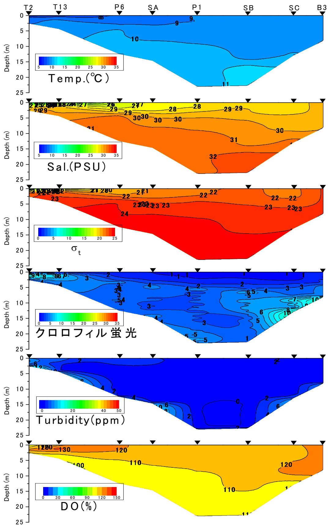
有明海湾奥西部海域の水質の断面分布 (2013年2月20日)
