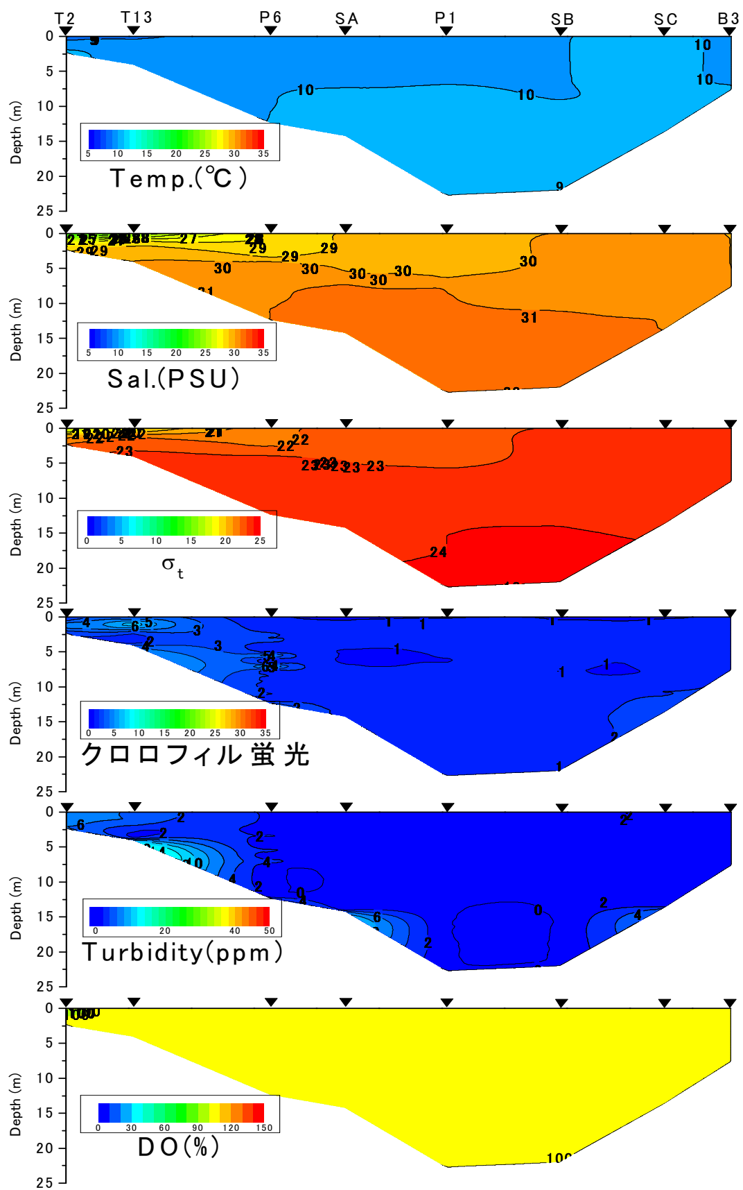
有明海湾奥西部海域の水質の断面分布（2013年2月5日）
