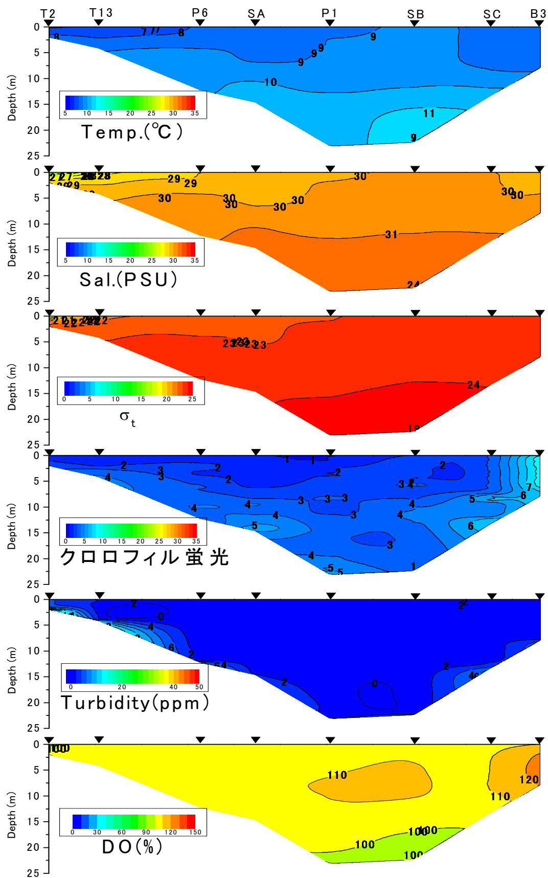
有明海湾奥西部海域の水質の断面分布（2013年1月21日）
