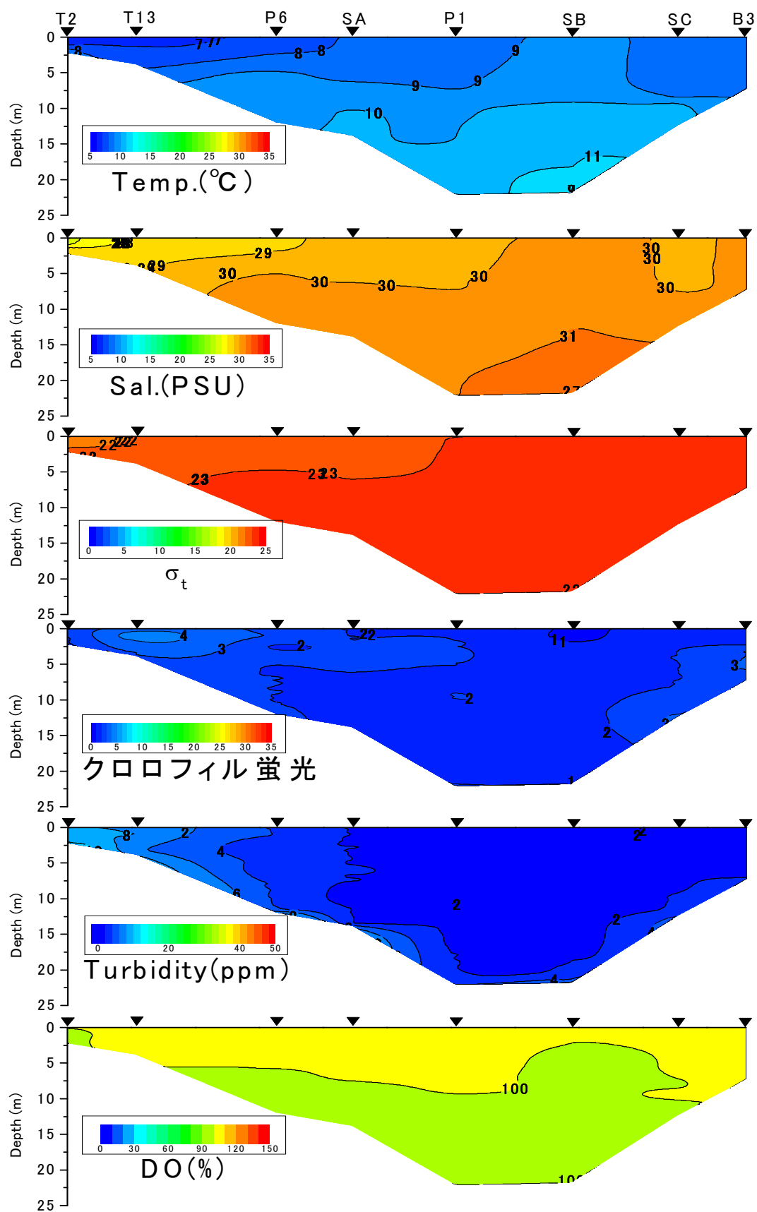
有明海湾奥西部海域の水質の断面分布（2013年1月7日）
