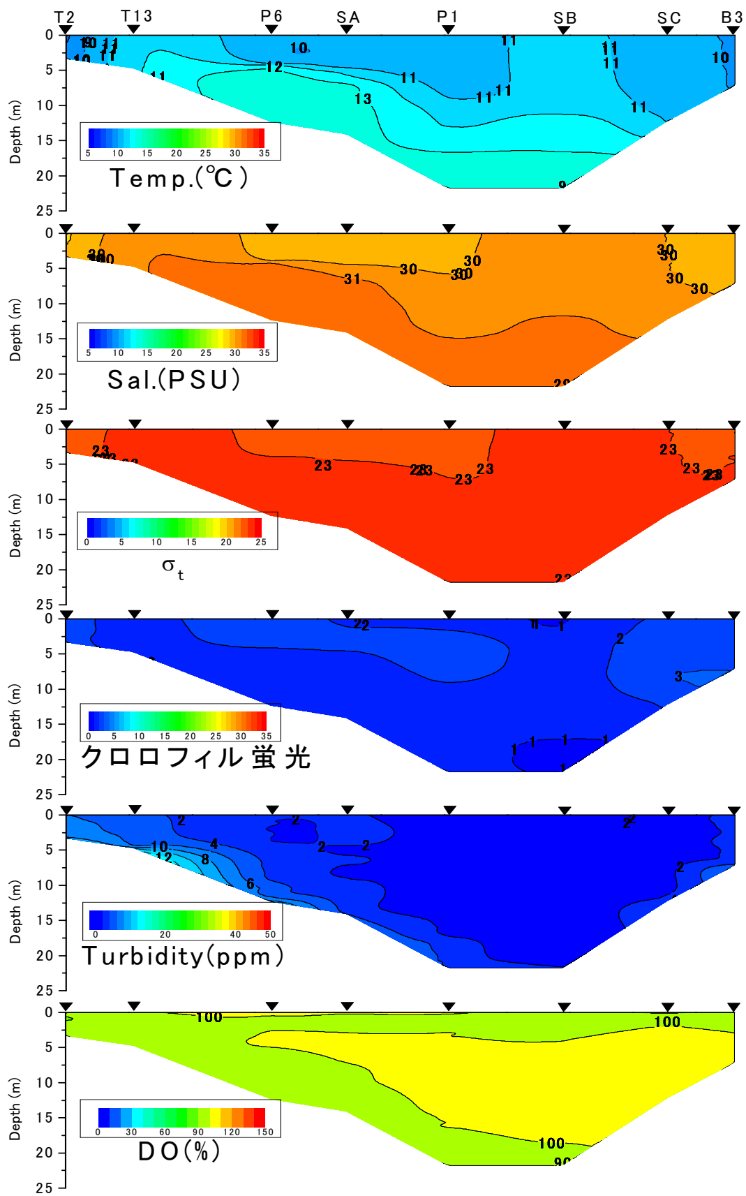
有明海湾奥西部海域の水質の断面分布 (2012年12月24日)
