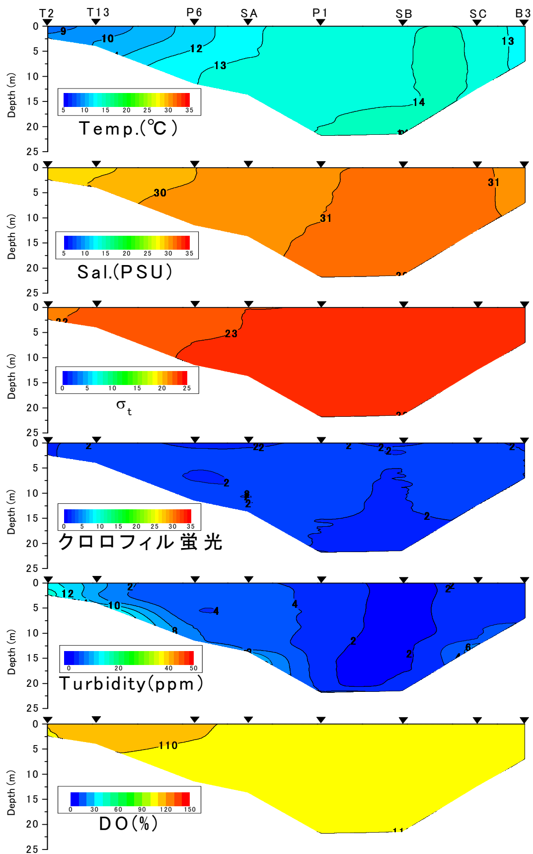
有明海湾奥西部海域の水質の断面分布（2012年12月10日）
