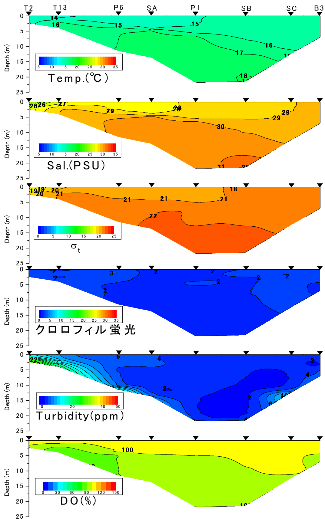
有明海湾奥西部海域の水質の断面分布（2012年11月21日）
