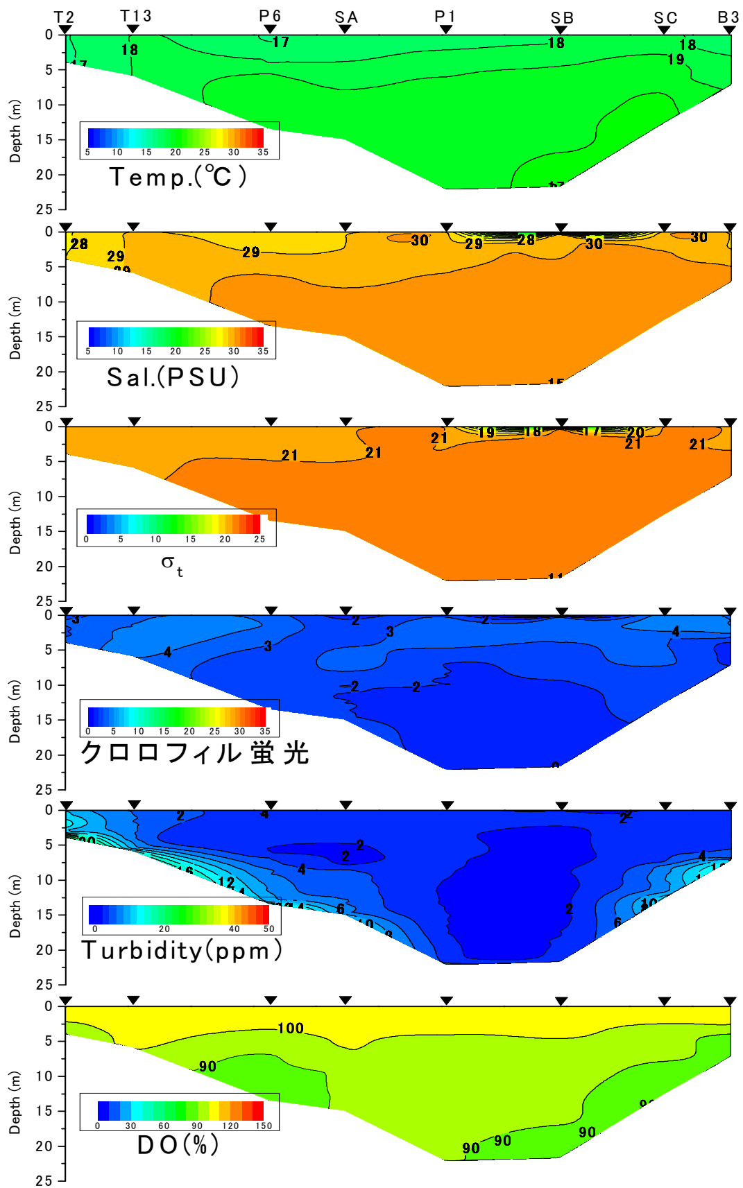
有明海湾奥西部海域の水質の断面分布 (2012年11月6日)
