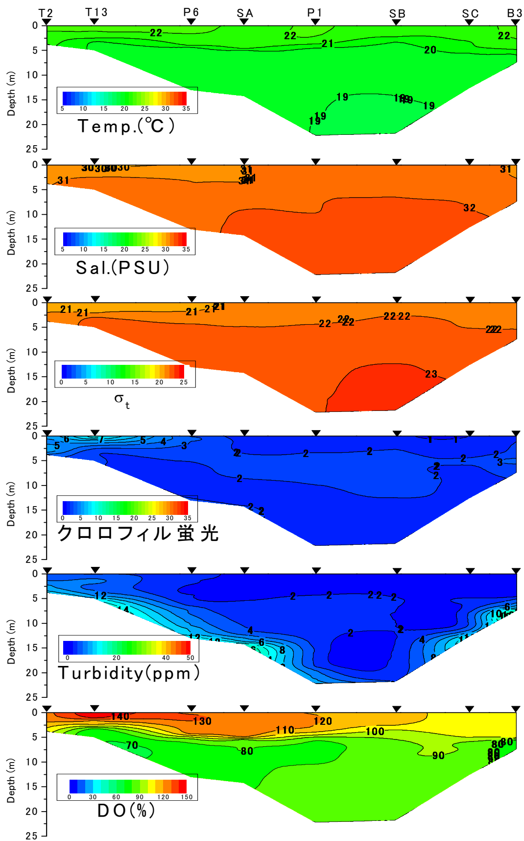
有明海湾奥西部海域の水質の断面分布（2012年5月30日）
