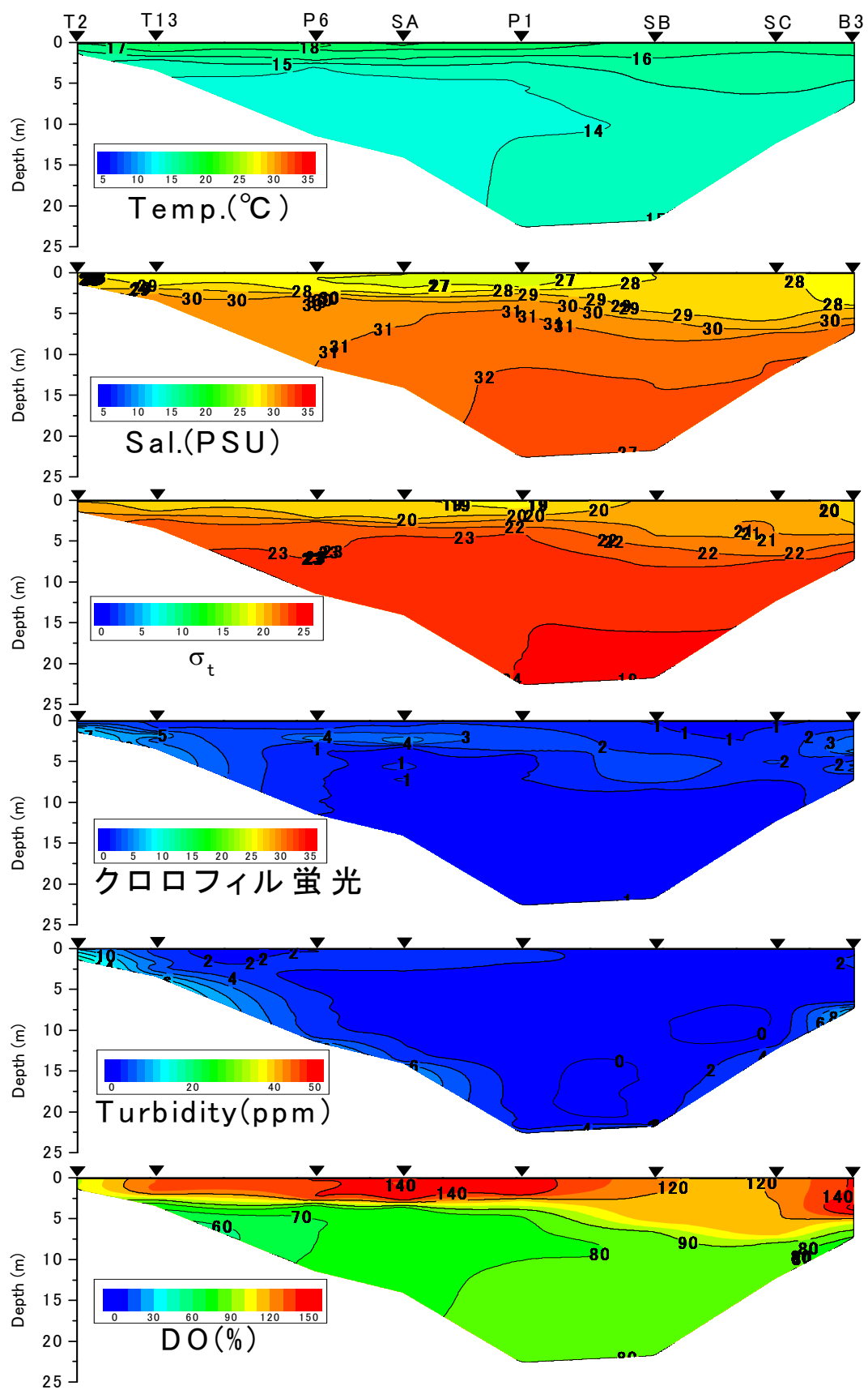
有明海湾奥西部海域の水質の断面分布（2012年4月16日）
