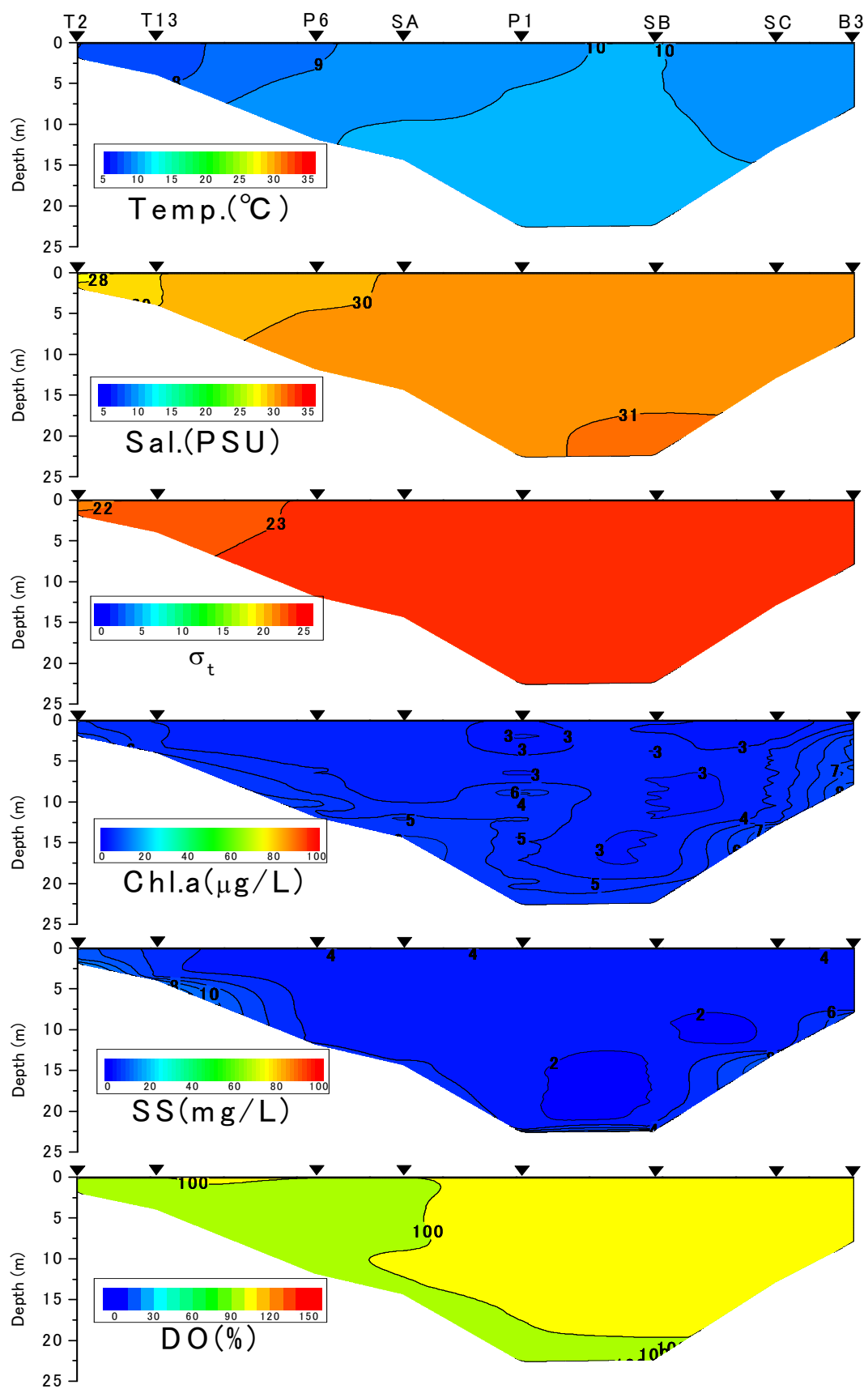
有明海湾奥西部海域の水質の断面分布（2012年1月18日）
