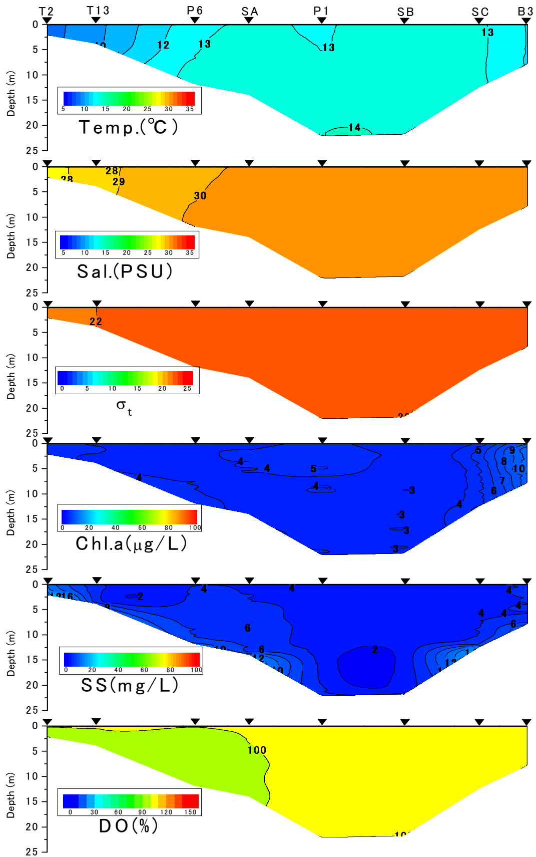
有明海湾奥西部海域の水質の断面分布 (2011年12月20日)
