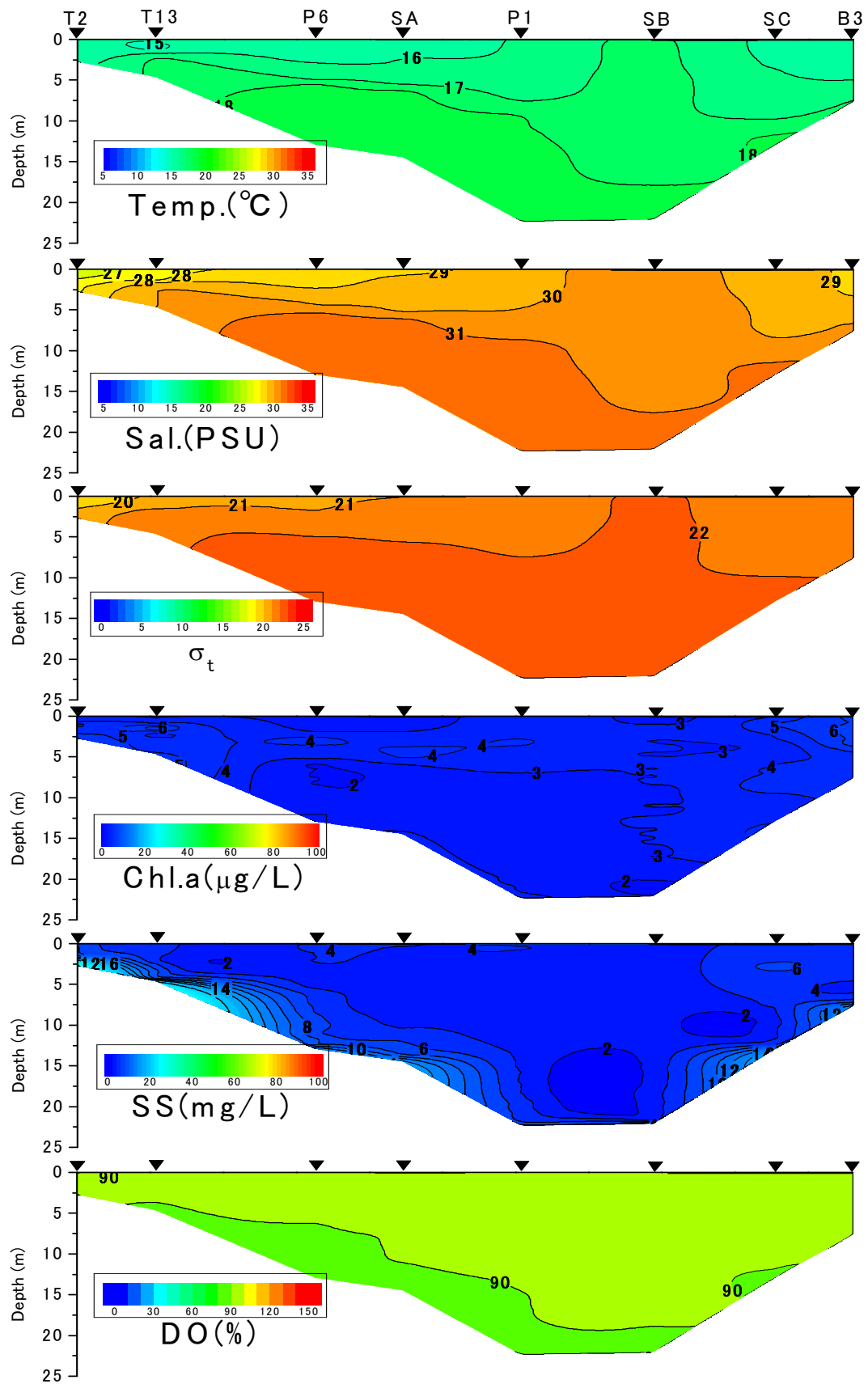
有明海湾奥西部海域の水質の断面分布（2011年12月4日）
