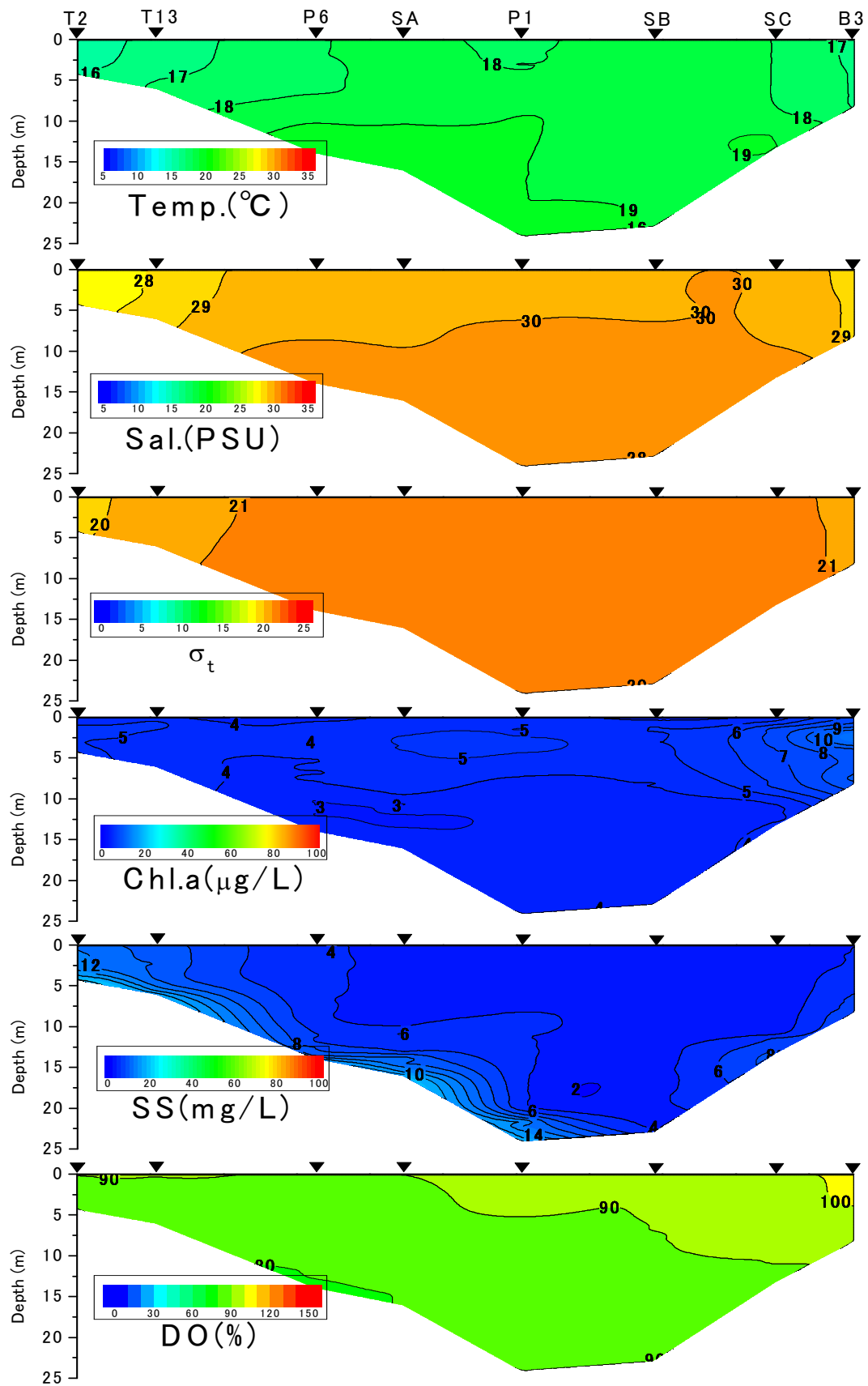
有明海湾奥西部海域の水質の断面分布（2011年11月24日）
