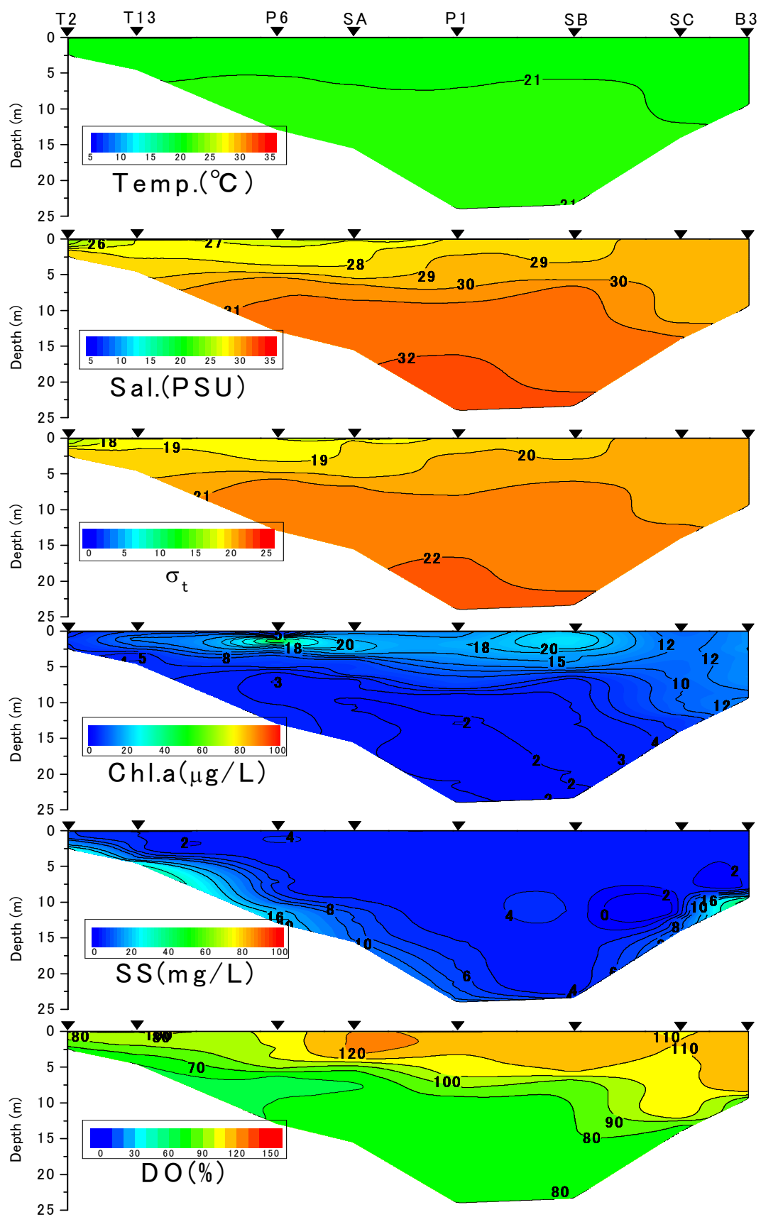
有明海湾奥西部海域の水質の断面分布（2011年11月7日）
