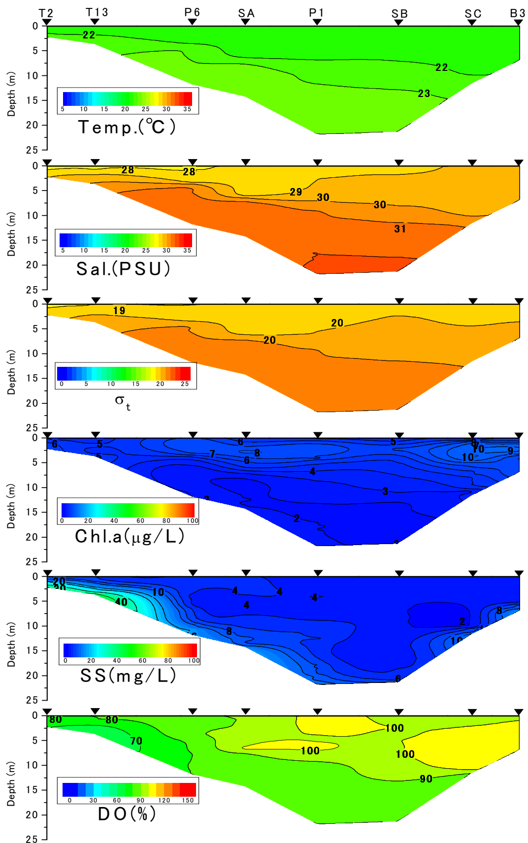
有明海湾奥西部海域の水質の断面分布（2011年10月23日）
