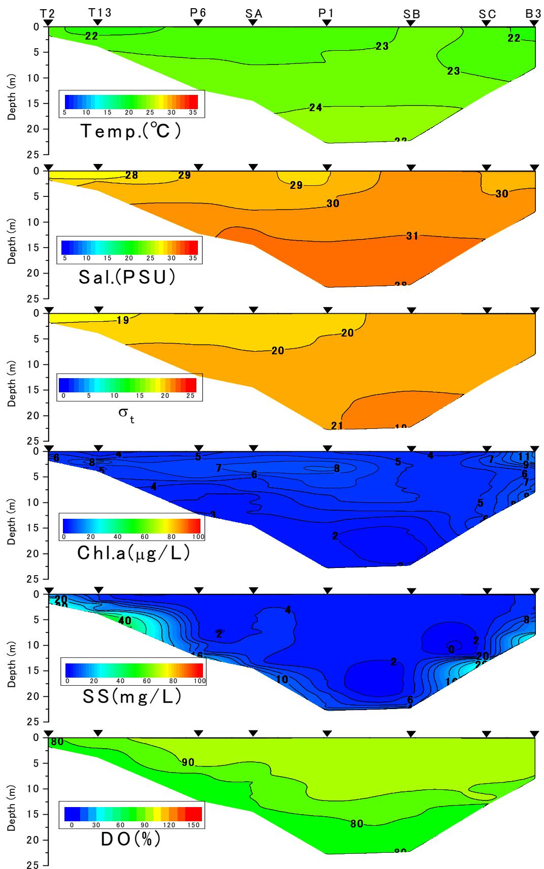
有明海湾奥西部海域の水質の断面分布（2011年10月6日）
