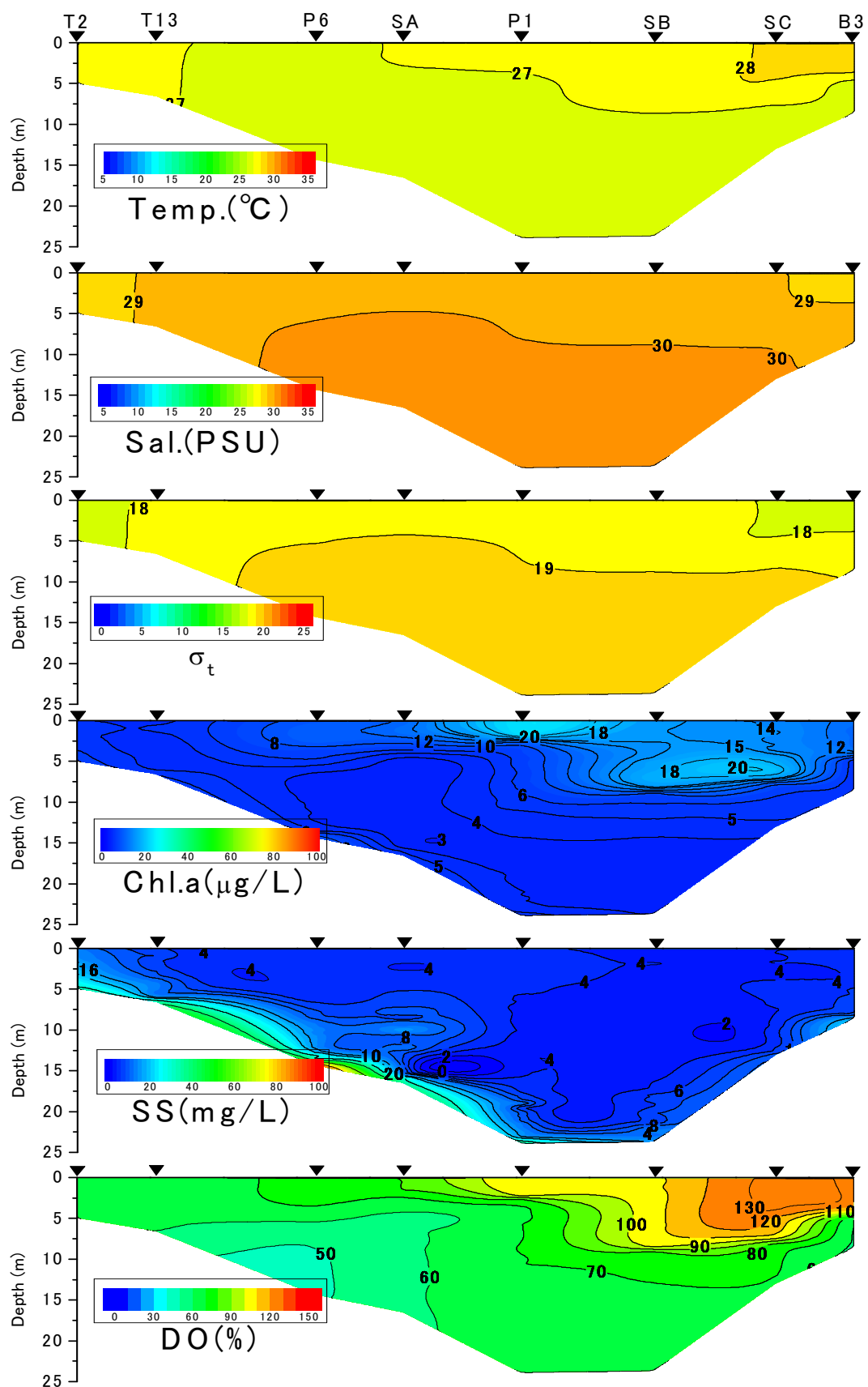
有明海湾奥西部海域の水質の断面分布（2011年9月14日）
