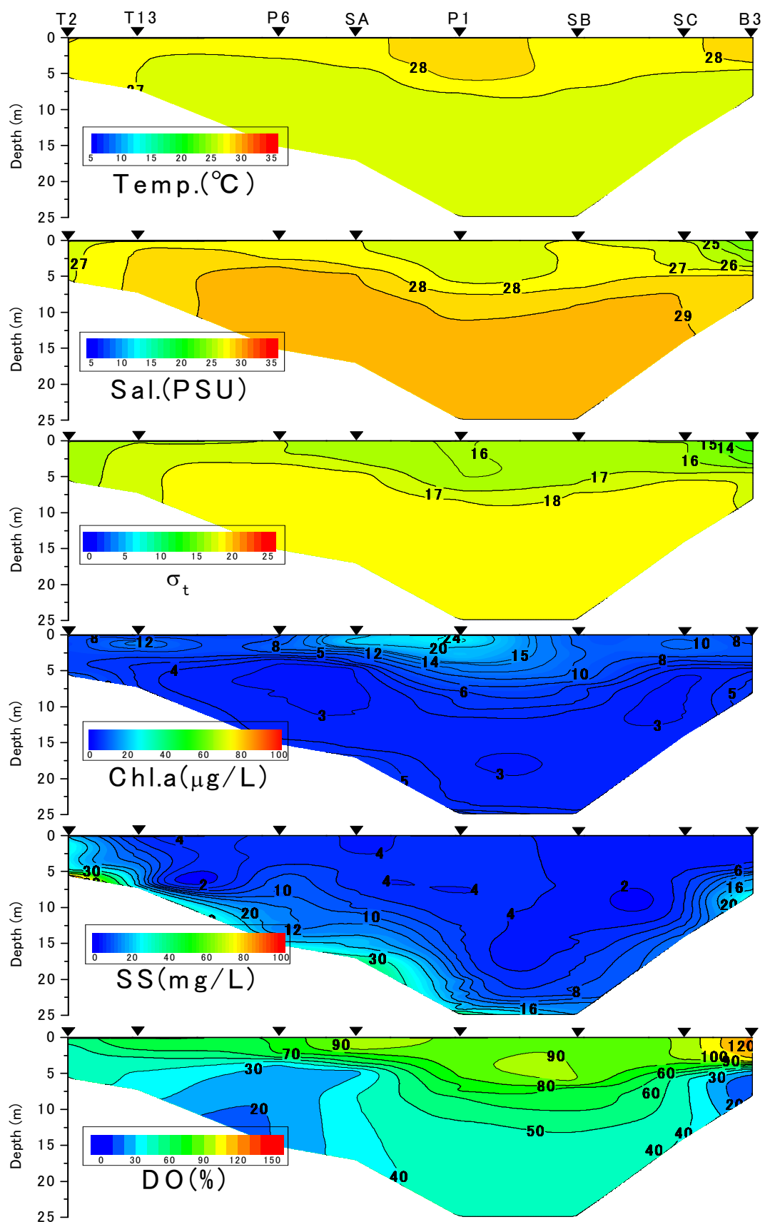
有明海湾奥西部海域の水質の断面分布（2011年8月31日）
