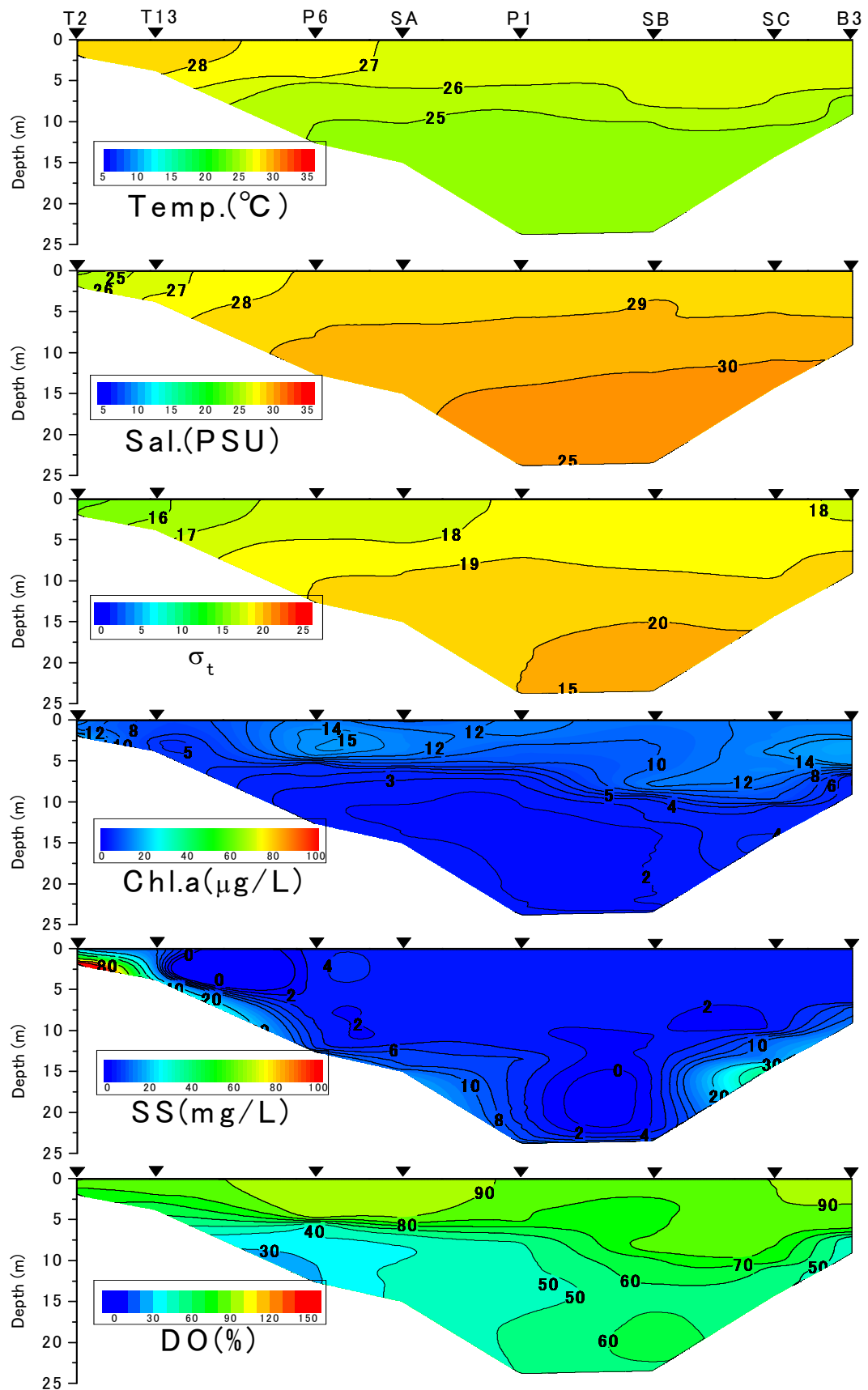
有明海湾奥西部海域の水質の断面分布（2011年8月9日）
