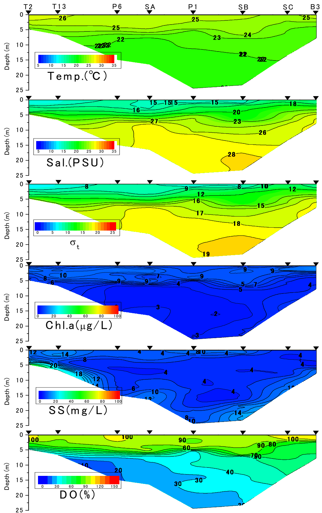
有明海湾奥西部海域の水質の断面分布（2011年7月5日）
