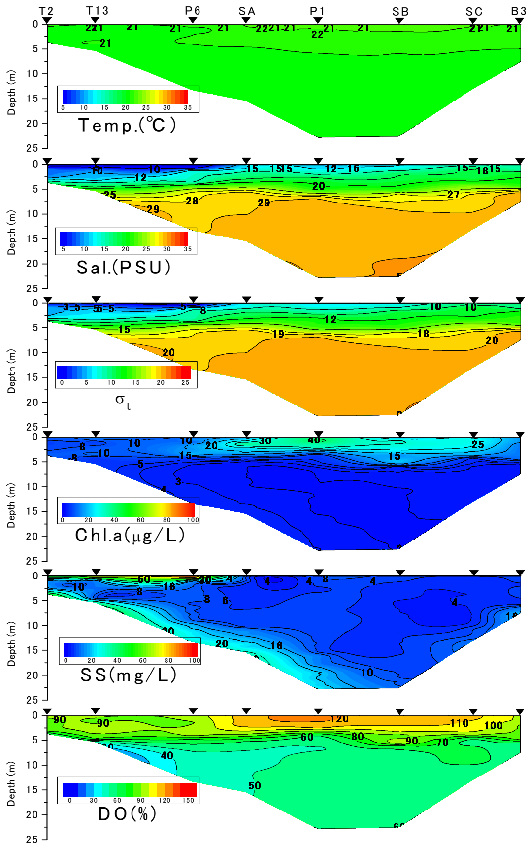
有明海湾奥西部海域の水質の断面分布（2011年6月21日）
